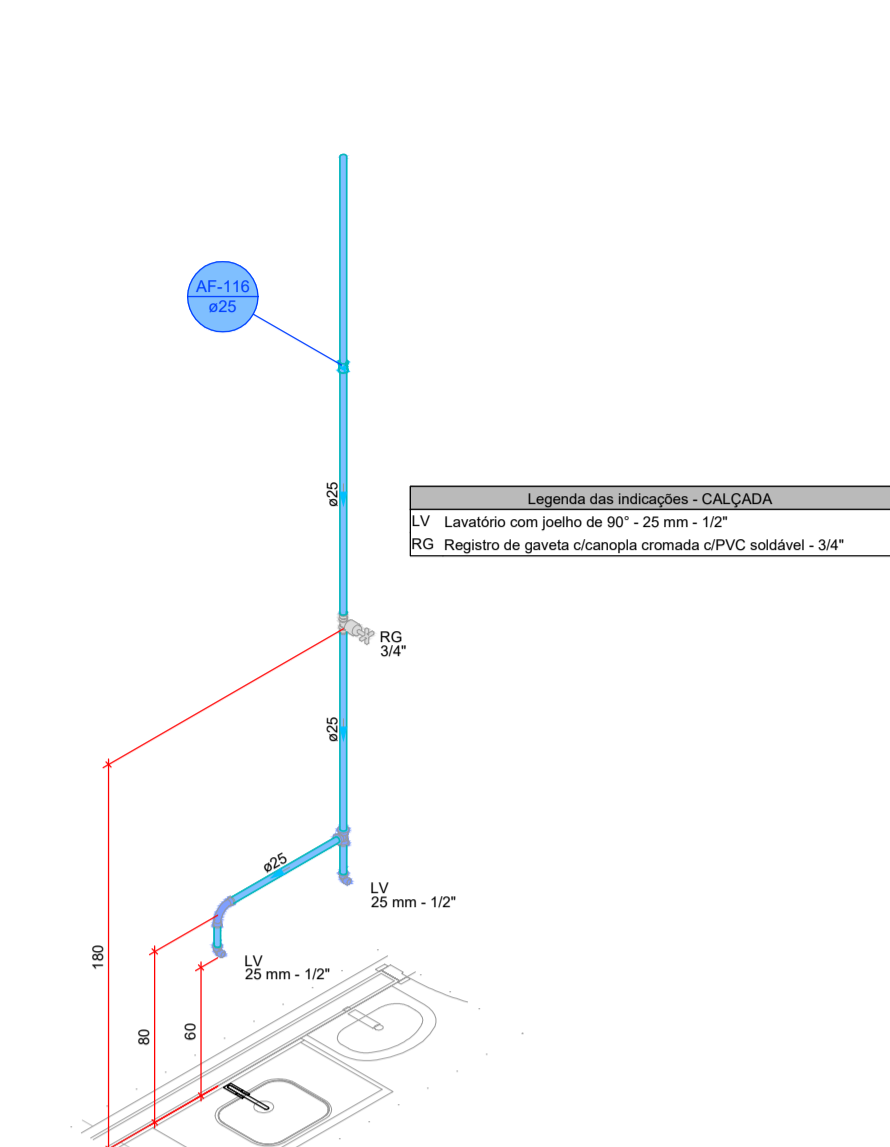
DETALHE HID-68 1:25
