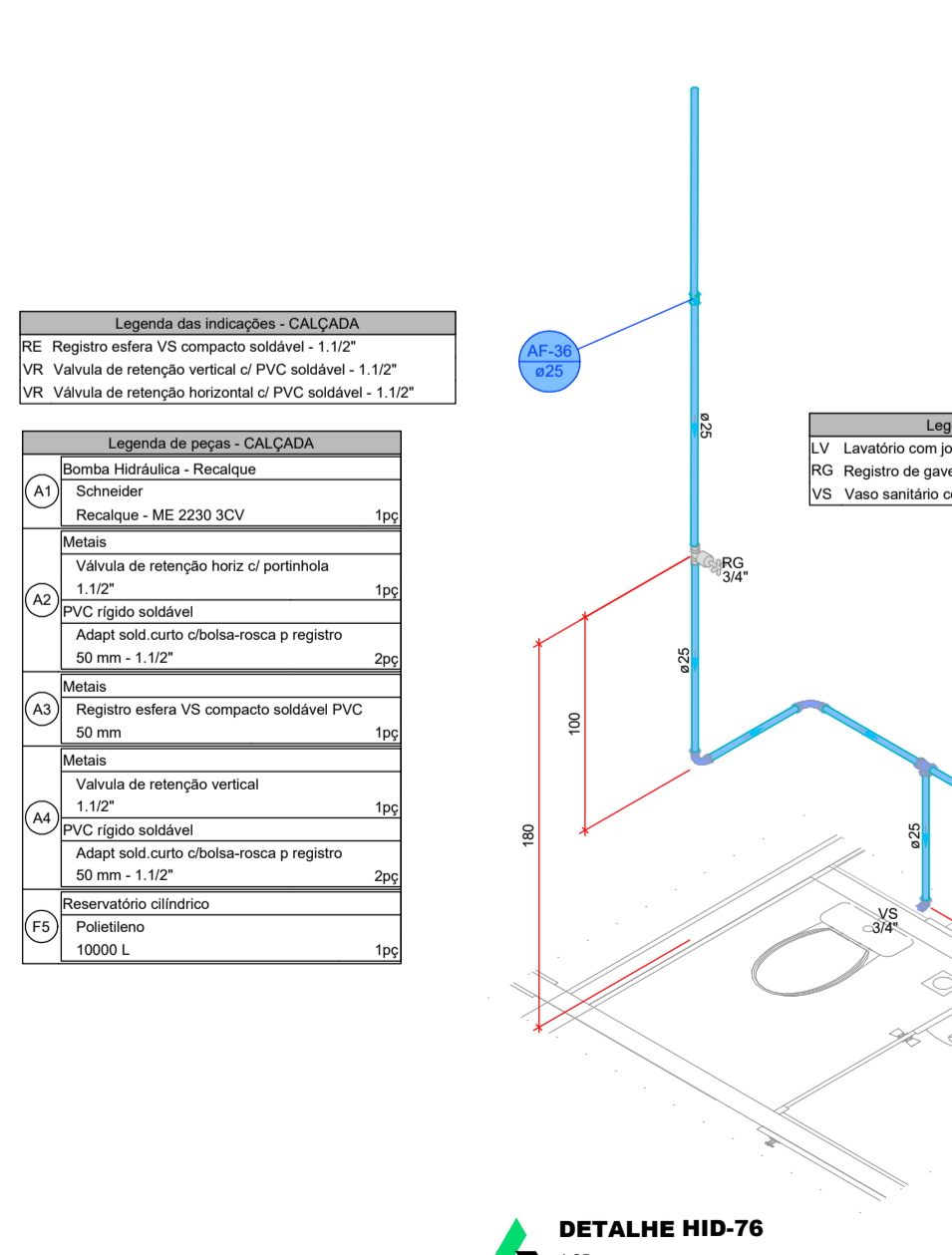
DETALHE HID-76 1:25
