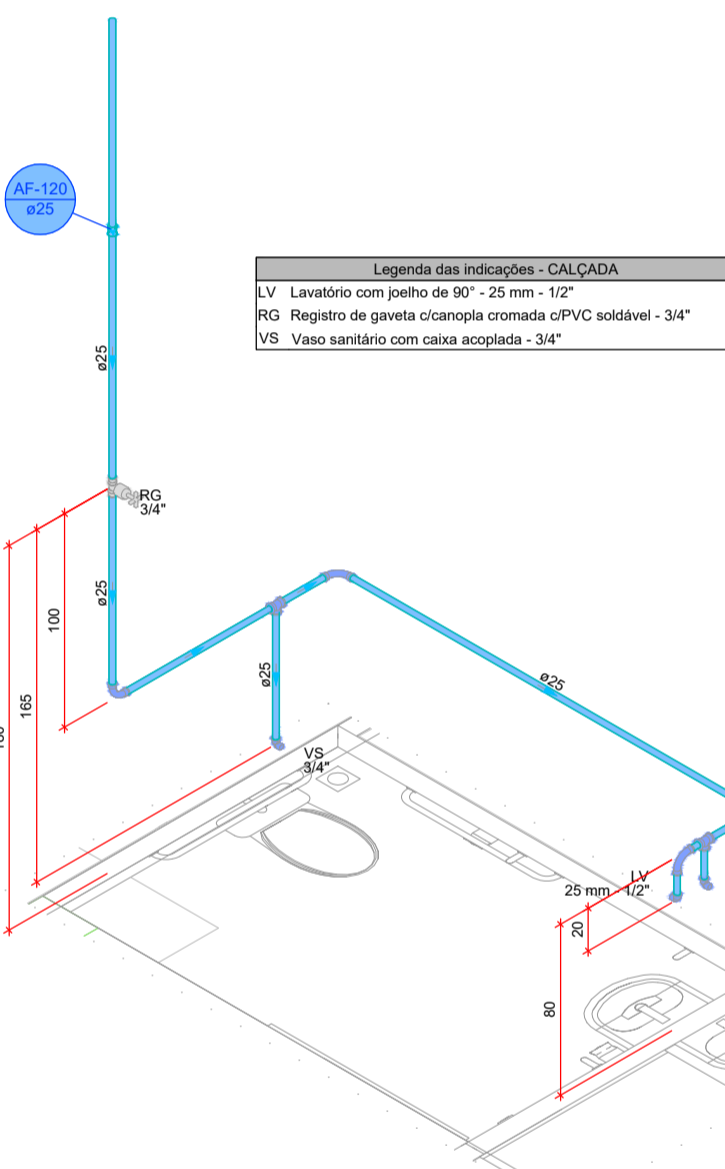
DETALHE HID-70 1:25
