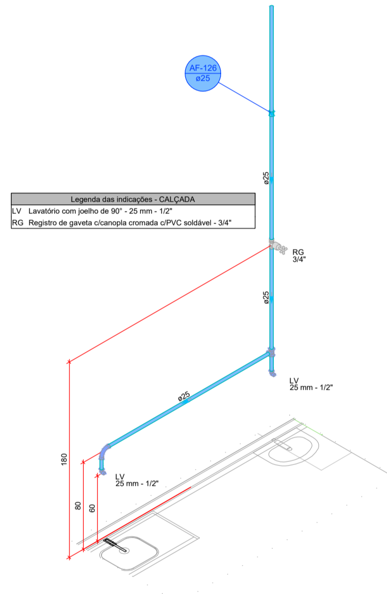
DETALHE HID-71 1:25
