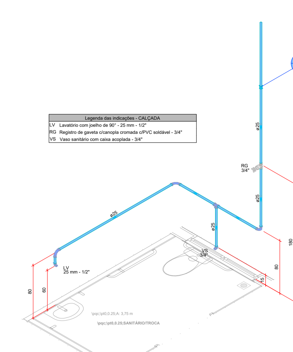
DETALHE HID-69 1:25
