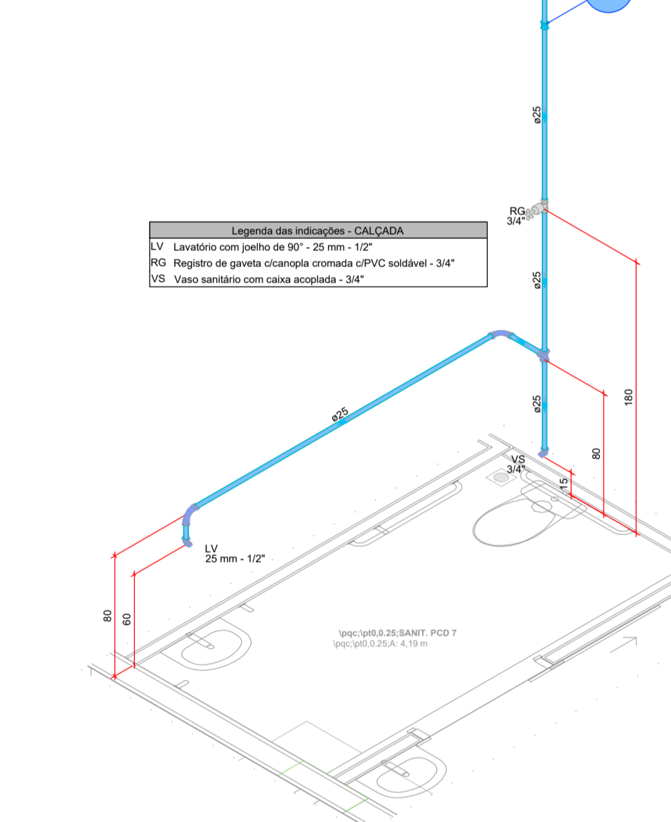
DETALHE HID-72 1:25
