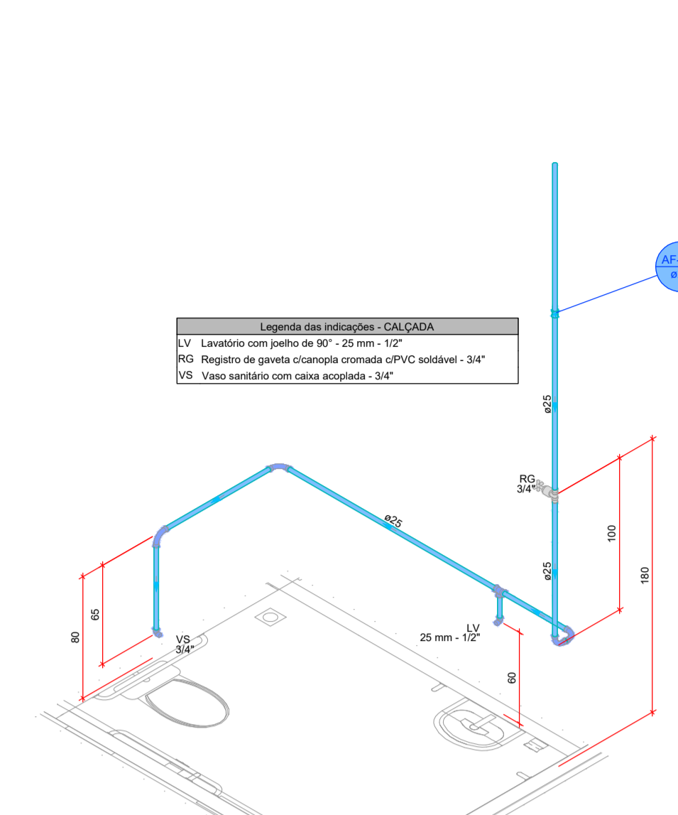
DETALHE HID-67 1:25
