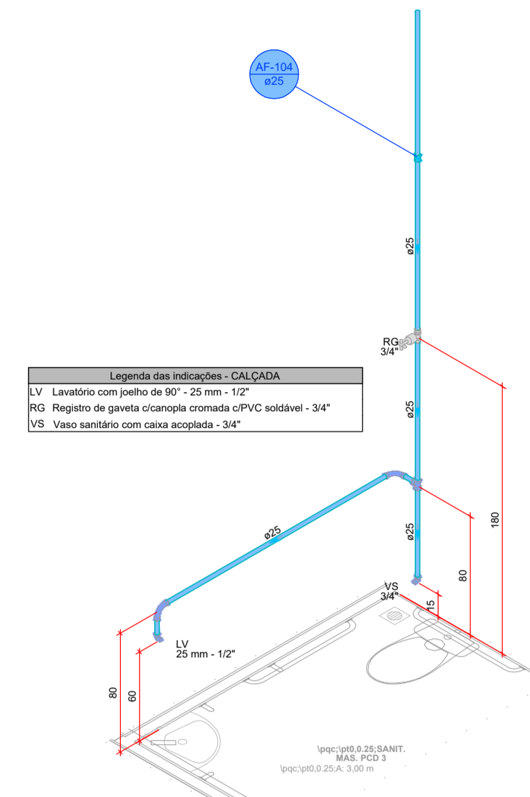
DETALHE HID-66 1:25
