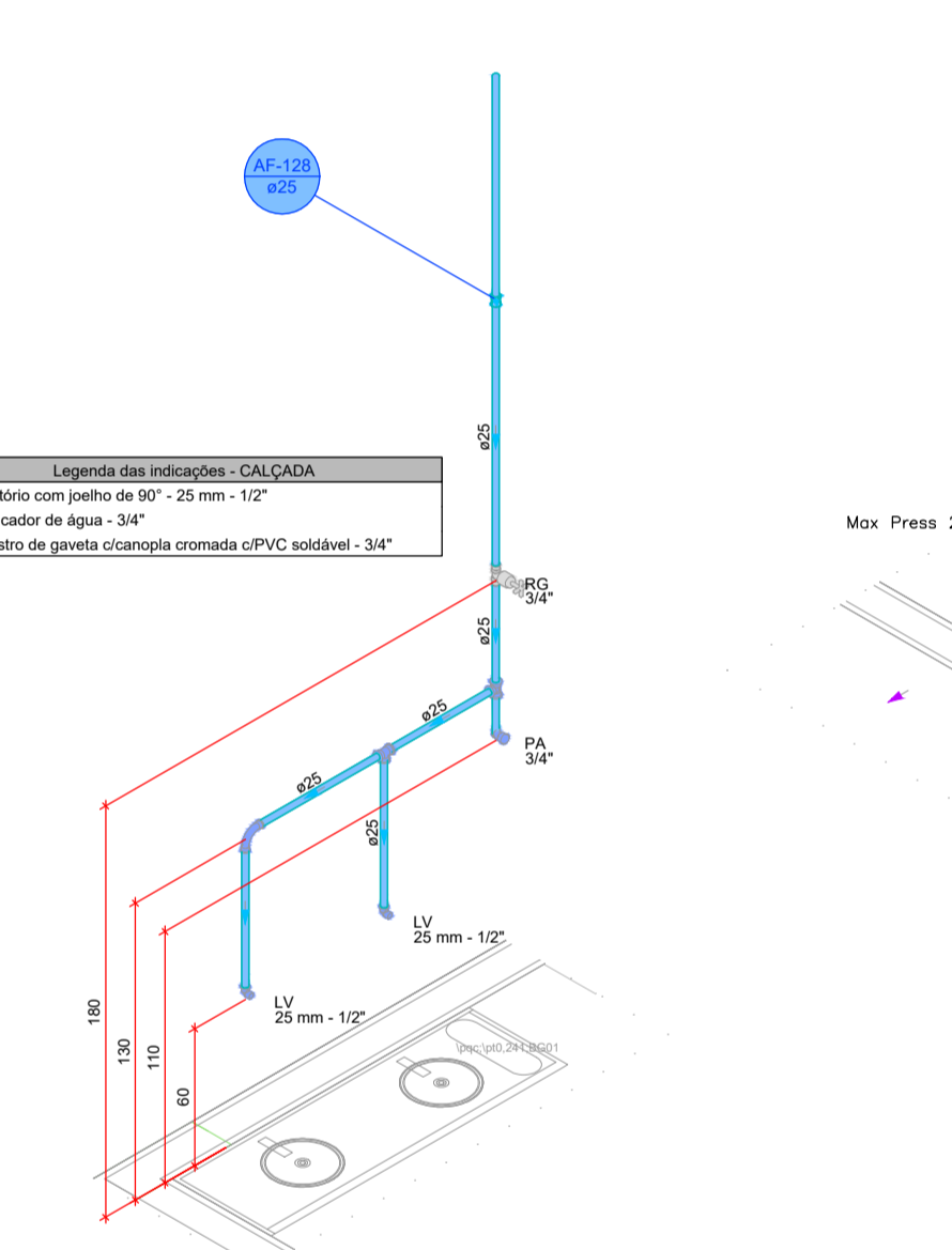
DETALHE HID-73 1:25
