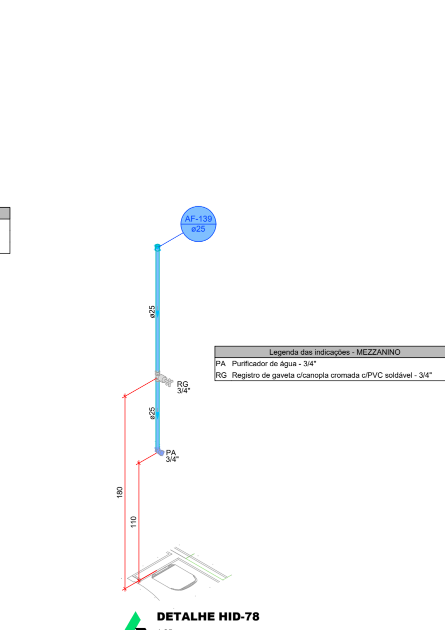
DETALHE HID-77 1:25
