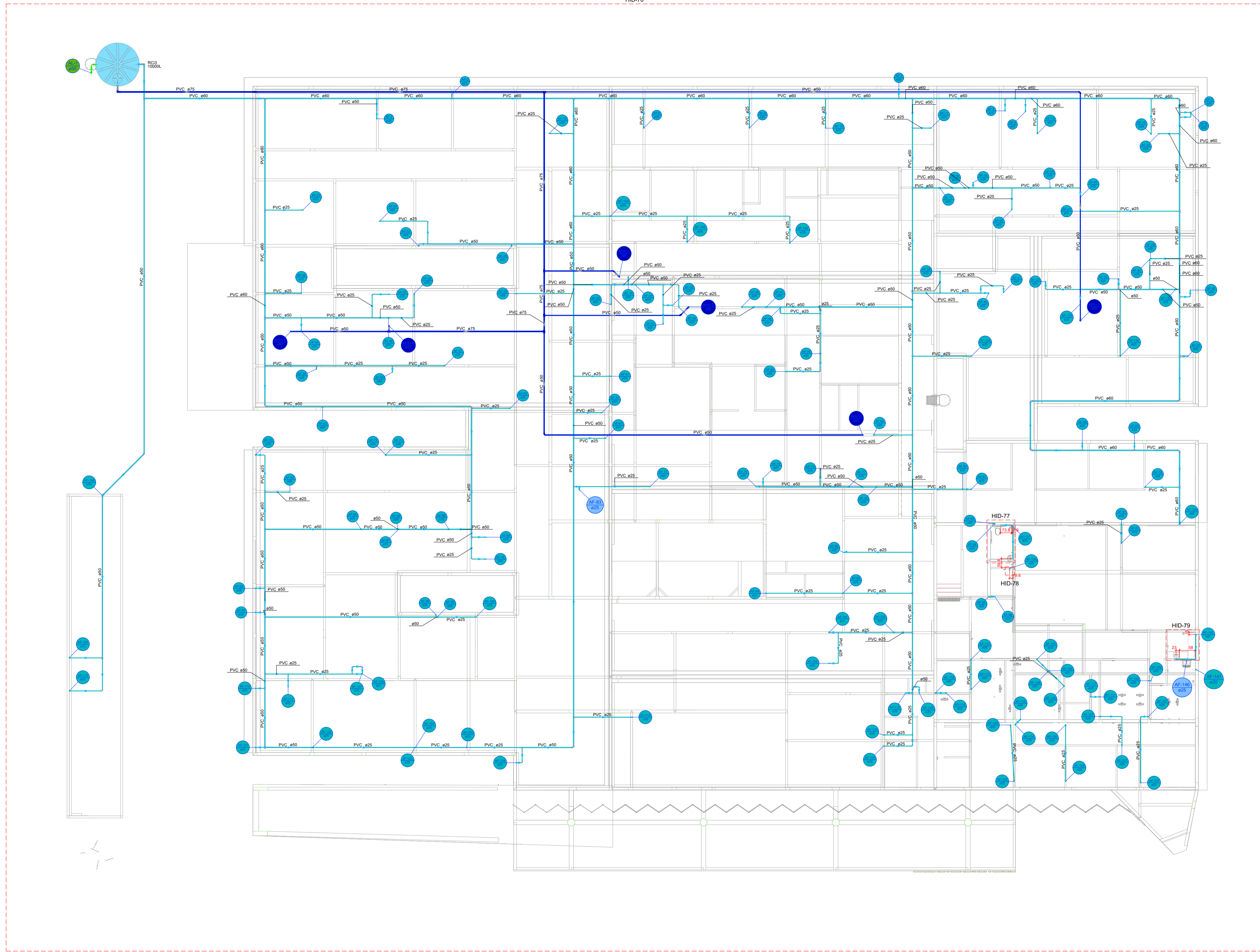
PLANTA - HIDRÁULICO - MEZANINO ESC. 1/100
