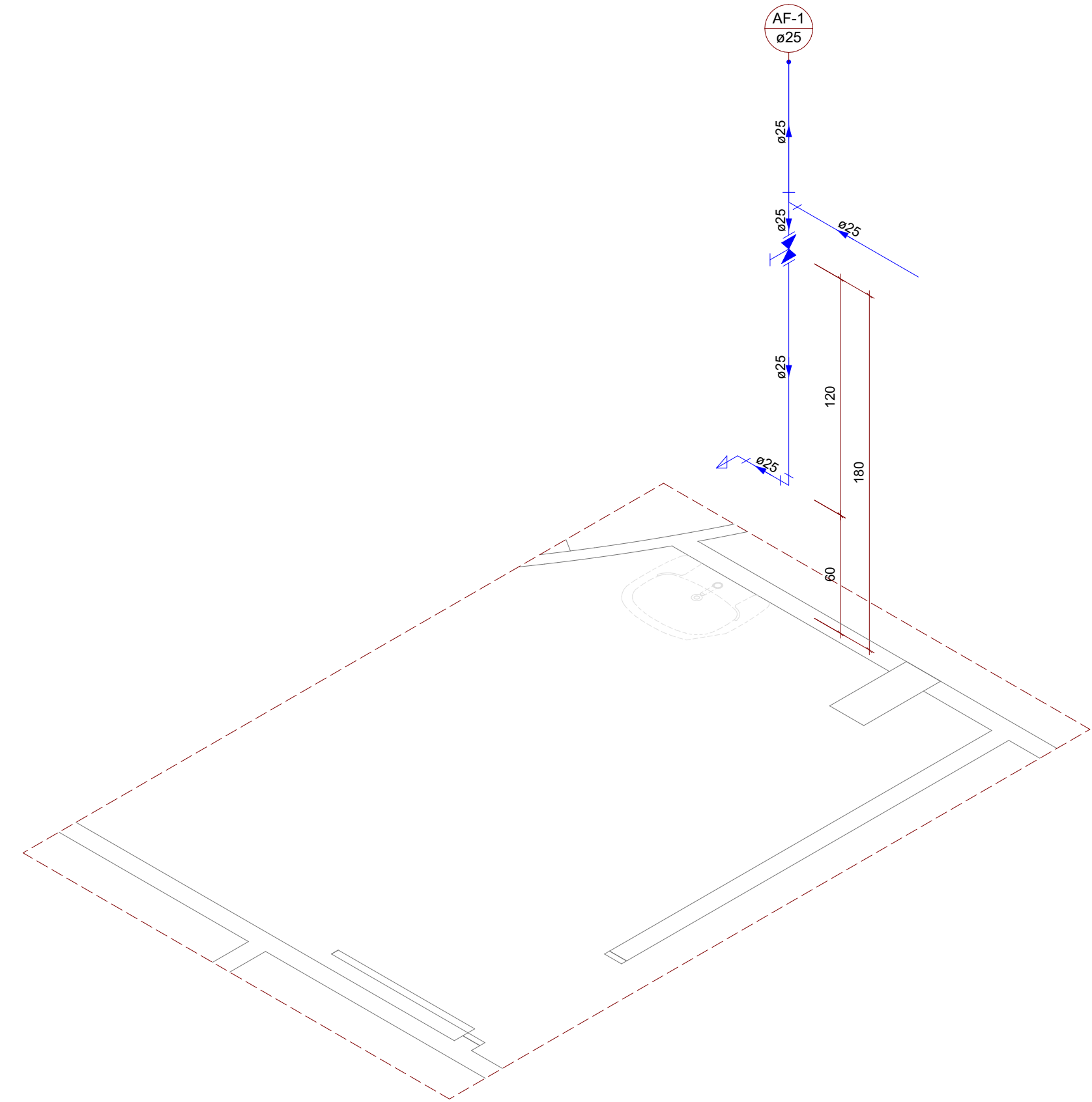
Isométrico: HID-1 Escala: 1:100
