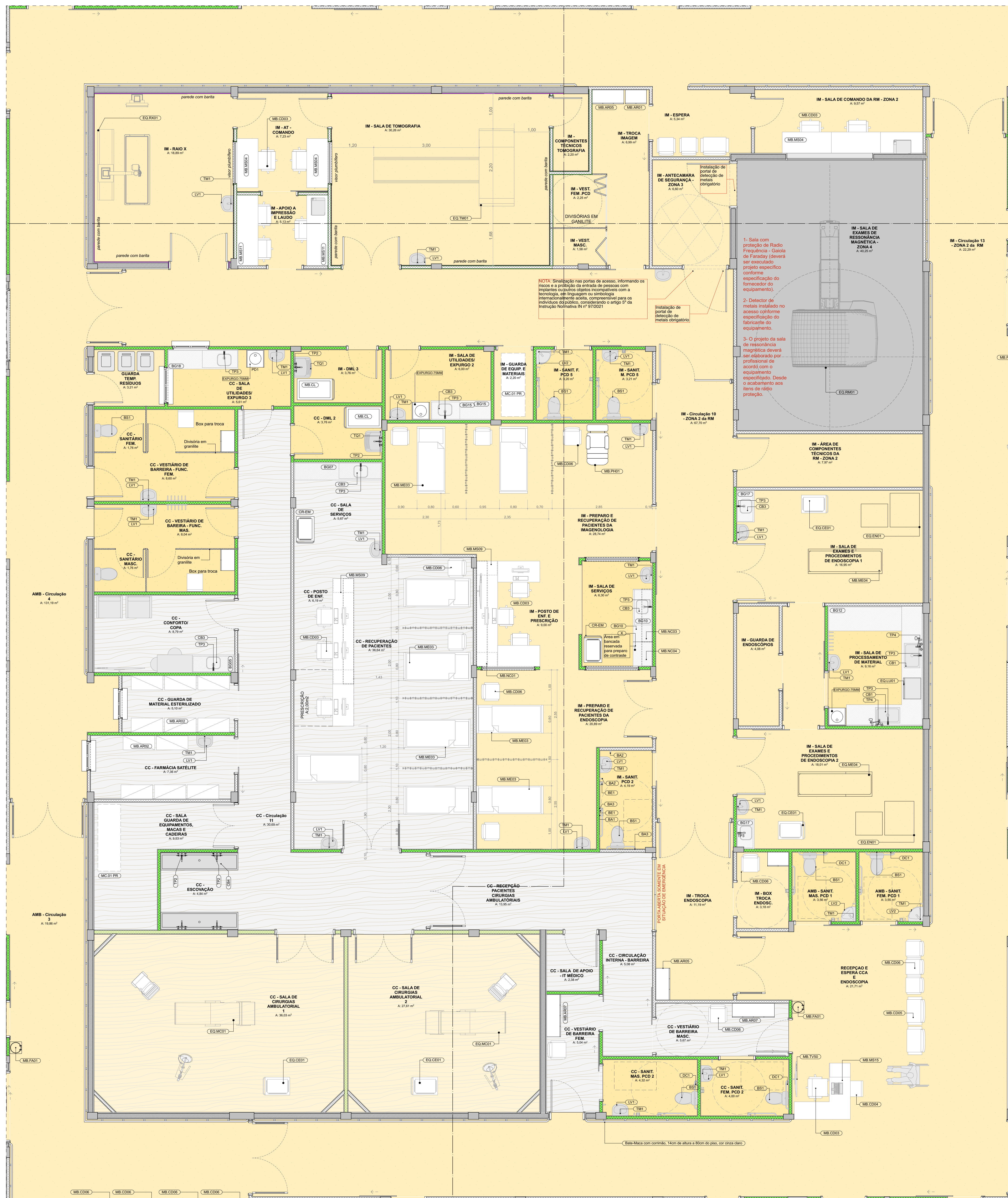
PLANTA DE LAYOUT TERREO Esc. = 1:50
