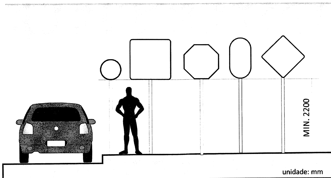
Figura 2 – Altura mínima livre das placas de solo a implantar.
