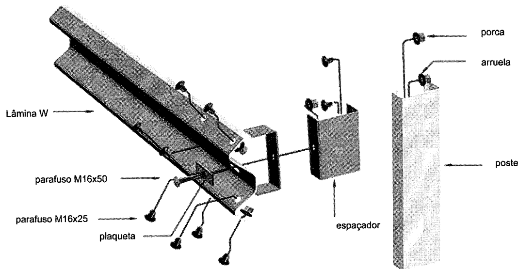
Figura 1 – Layout de implantação – Defesa semi-maleável simples.
